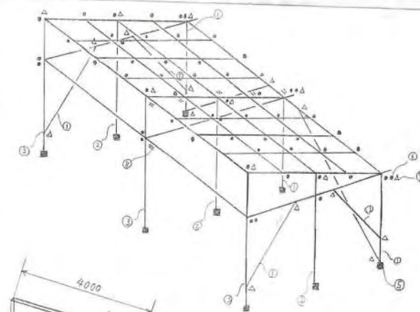
休憩所の設計単管骨組み
